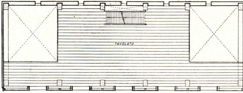
PIANTA DEI PIANI III° IV° V° - SEZ. D-D E-E F-F
