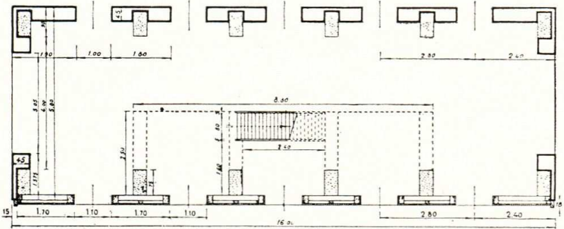
PIANTA DEL PIANO TERRENO - SEZ. A-A
