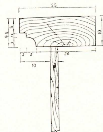
PARTICOLARE DEL DAVANZALE
