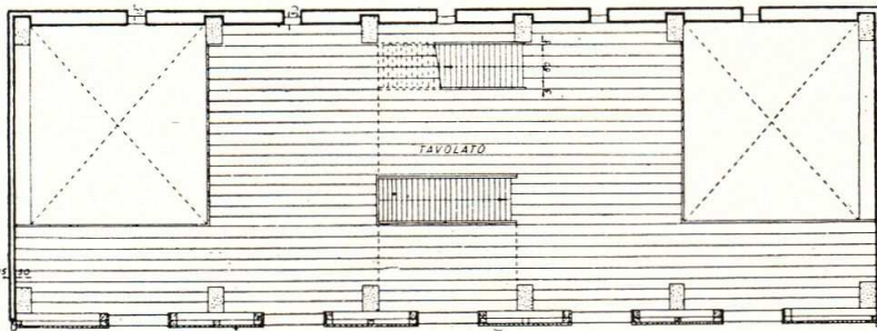
PIANTA DEL II° PIANO - SEZ. C-C
